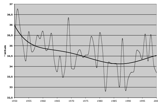
Fig. 10 – Latitude atteinte par les AMP
