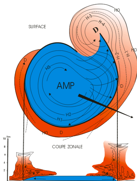
Fig. 6 – Anticyclone Mobile Polaire (HN) surface et coupe verticale rouge : chaud et cyclonique bleu : froid et anticyclonique
