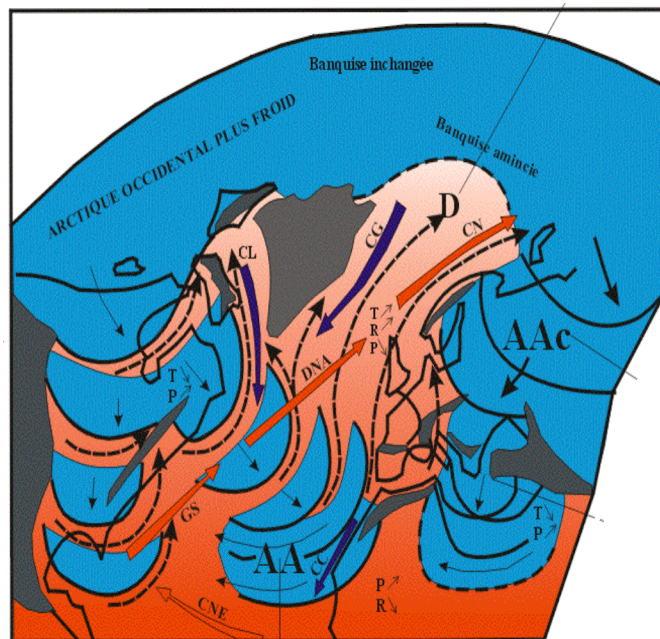
Fig. 16 – Unité Nord-Atlantique → mode de circulation rapide depuis 1970s T : température, P : pression, R : pluie
