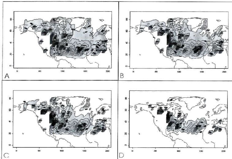
Fig. 7 : AMP américano-atlantiques en fonction de la pression moy. annuelle
