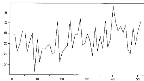
Fig. 12 – Latitude atteinte par les dépressions
