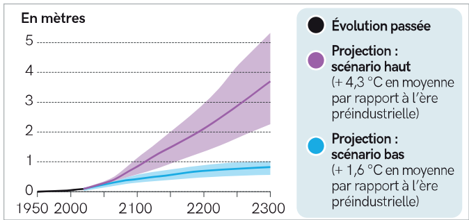
D'après le rapport du GIEC sur l'océan et la cryosphère, et Le Monde, 2019
