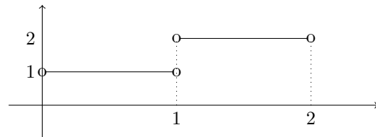
Une fonction non constante mais de dérivée identiquement nulle
