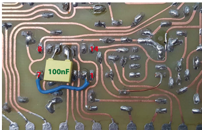
Modifs pour adapter le SSM2056 a la place du SSM2050
