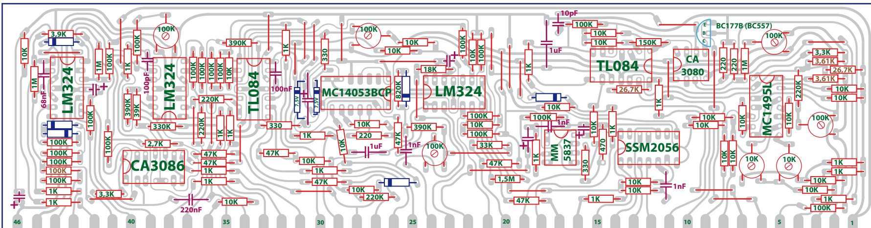
Modifs pour adapter le SSM2056 a la place du SSM2050
