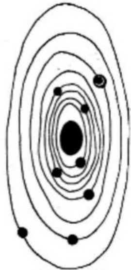
Fig. 2 : Le Système Solaire
