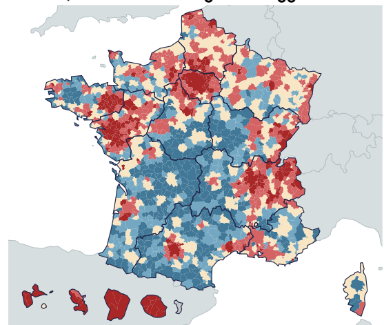
Taux de variation annuel de la population dû au solde naturel entre 1999 et 2013
