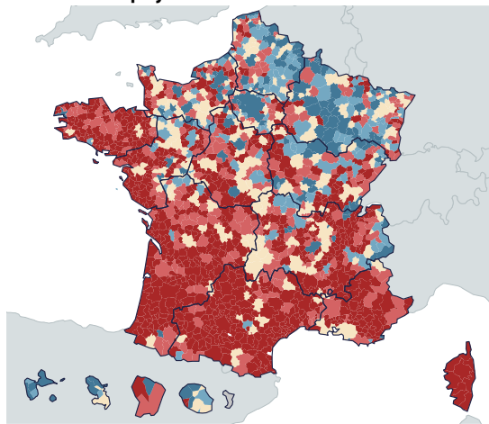
Taux de variation annuel de la population dû au solde migratoire entre 1999 et 2013
