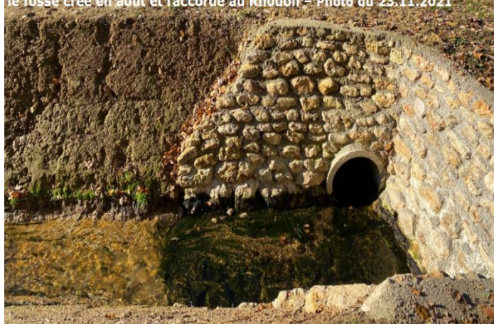
Buse de rejet des eaux épurées de la STEP du Mesnil-St-Denis dans le fossé crée en août et raccordé au Rhodon - Photo du 23.11.2021
