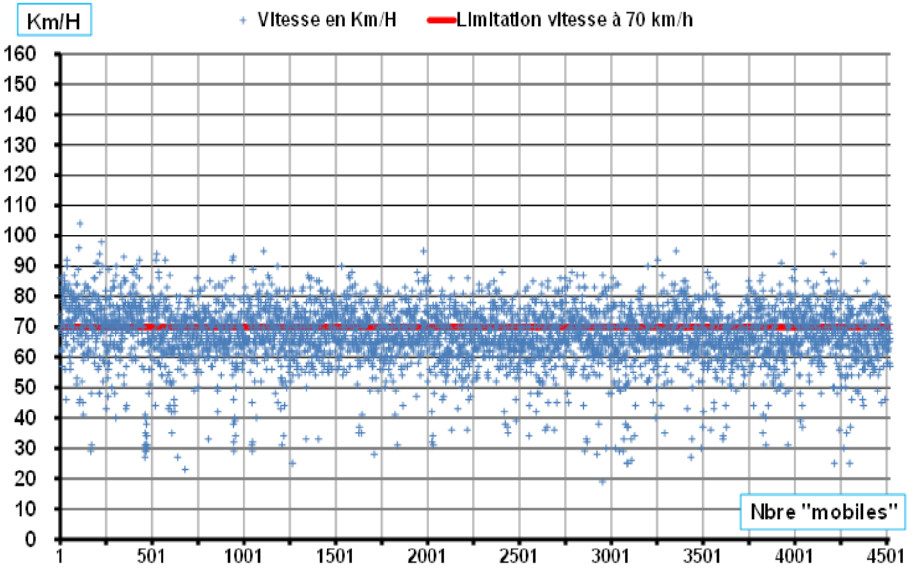
Répartition des vitesses mesurées pour la catégorie PL Période du jeudi 11 juin (0H) au mercredi 24 juin 2015 (24H)
