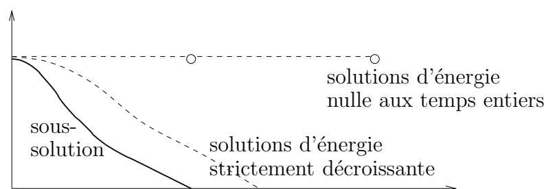
FIGURE 5. Construction de contre-exemples à l’unicité
