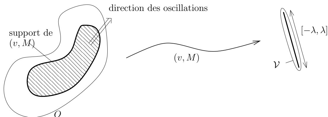
FIGURE 3. Ondes localisées à grande fréquence, d'après la proposition 3.2.
