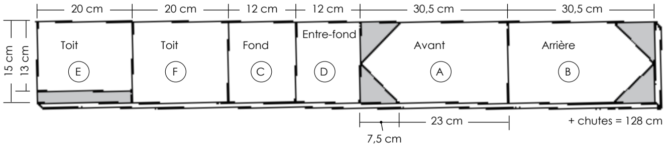
Plan de coupe
