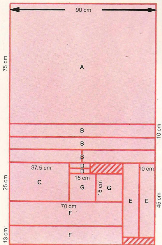
3. Plan de coupe du tablier d'hôtesse : A jupe; B bretelles (3); C bavette; D passants (2 de 12,5 x 4 cm); E ceinture (2); F volant (2); G poches (2).
