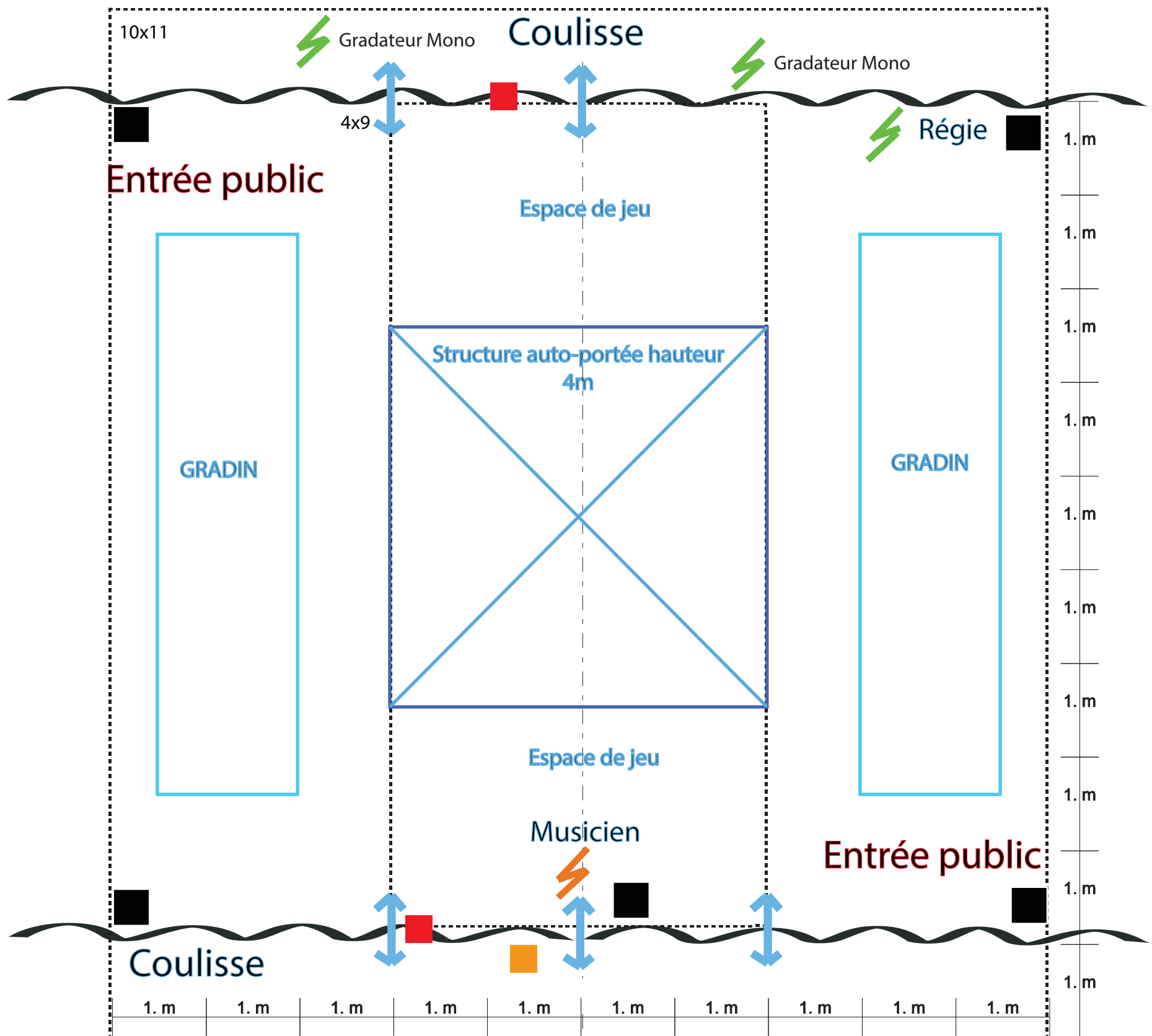
plan générique de principe ech. 1/50è
