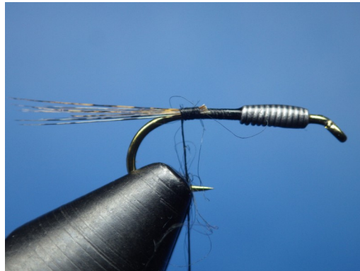
1. Après avoir fixé l'hameçon, enrouler le fil de plomb selon les lestages désirés et fixer les cerques en fibres de coq pardo.
