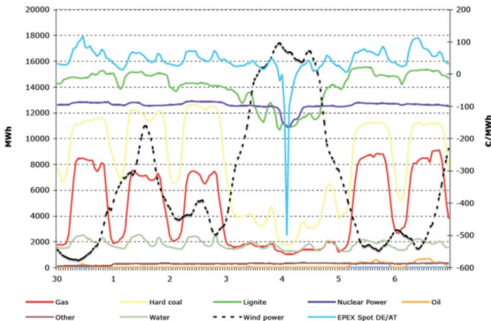
Schéma n° 9 Réaction de différentes technologies de production en Allemagne aux prix de l'électricité négatifs le 4 octobre 2009
