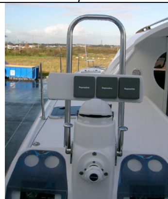
Console inox électronique sur tube inox bâbord Electronic console on an S/S tube portside
