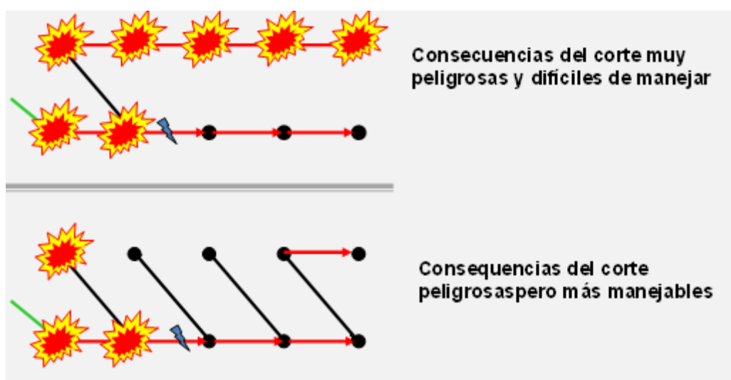
Figura 55: Selección de una secuencia de disparo que reduce el riesgo de consecuencias de un corte
