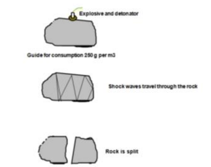
Figura 59: Taqueo de un bloque mediante un parche adosado al mismo
