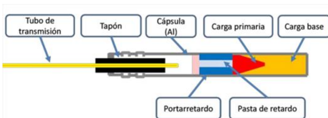
Figura 14: Esquema de un detonador no eléctrico
