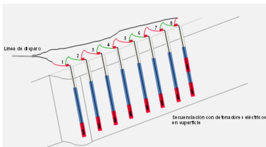
Figura 26: Secuencia en superficie con detonadores eléctricos
