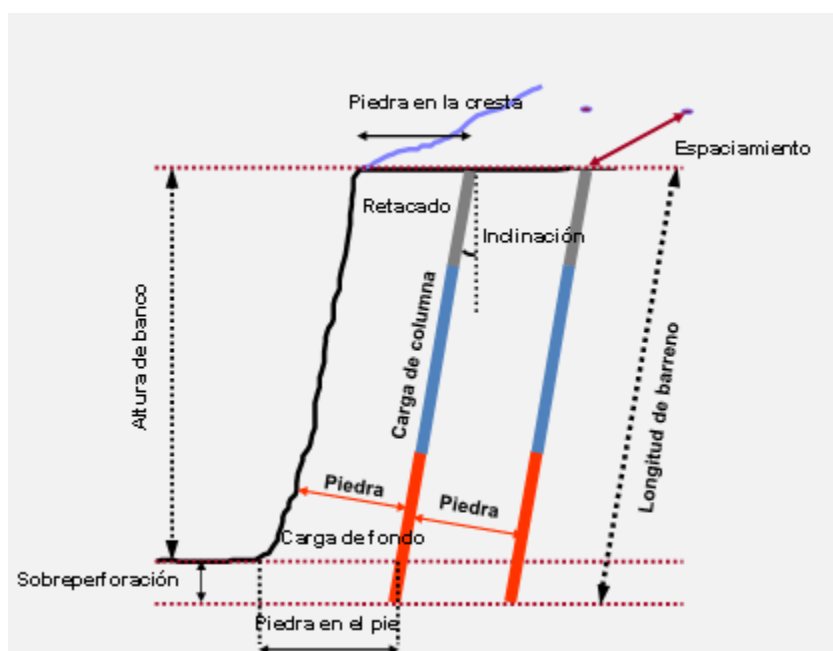
Figura 49: Esquema de los parámetros geométricos de diseño de una voladura en banco
