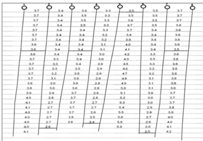
Figura 42: Vista frontal de una perforación real, obtenida mediante sonda electrónica
