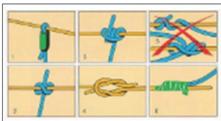
Figura 18: Posibles uniones de cordón detonante
