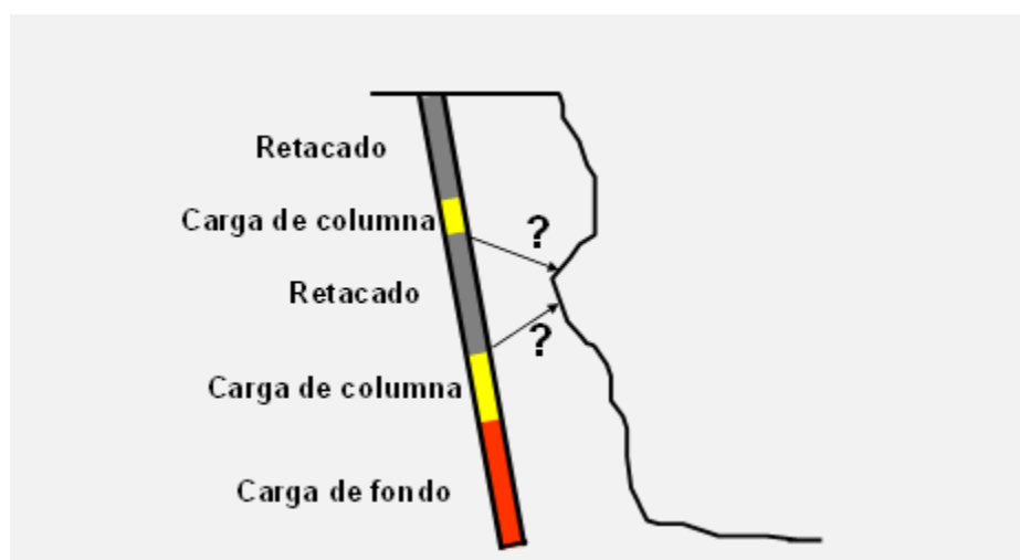
Figura 56: Uso de un retacado intermedio para evitar una piedra reducida en el perfil del banco
