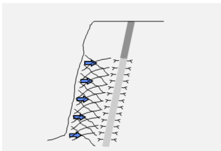
Figura 47: Reflexión de las ondas en la cara libre del frente del banco
