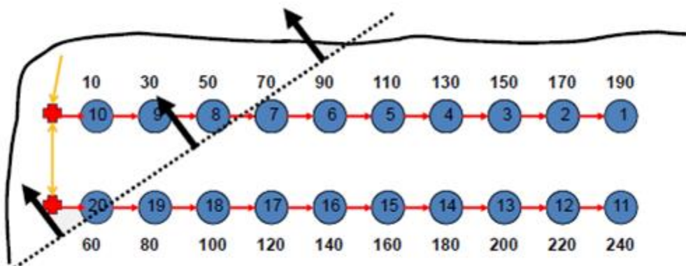
Figura 54: Dirección de la salida de la voladura mediante secuenciación de los barrenos
