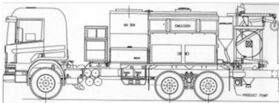
Figura 12: Esquema de un MEMU
