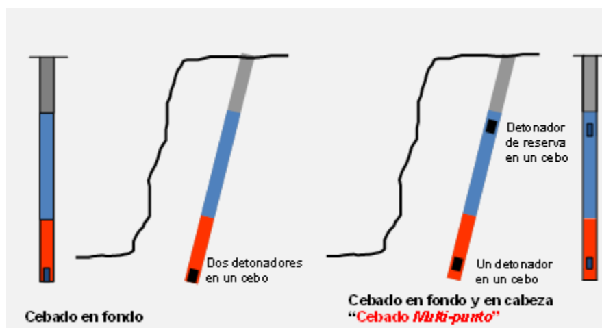
Figura 24: Esquema de iniciación en fondo de barreno
