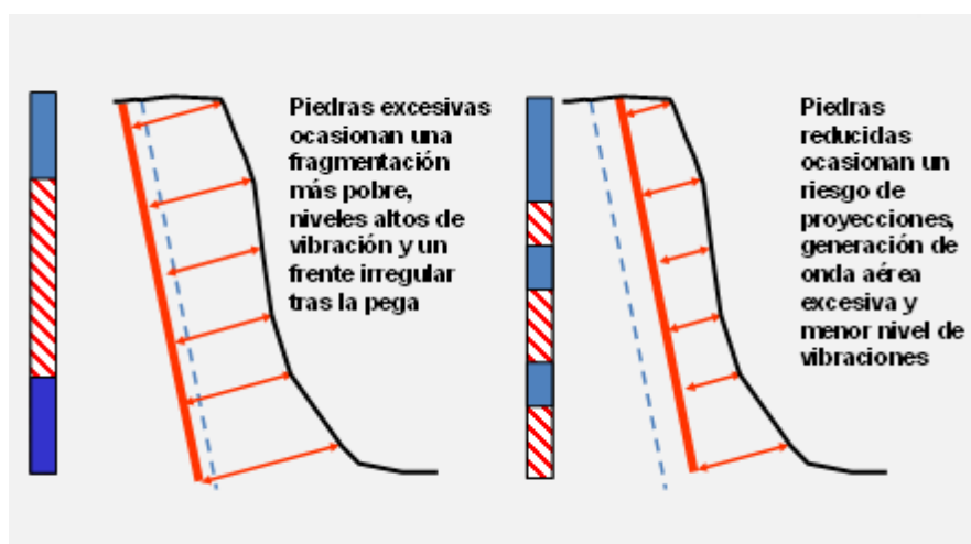
Figura 50: Consecuencias posibles de piedras incorrectas en la voladura
