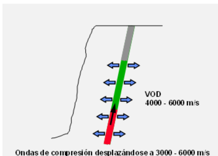
Figura 46: Esquema de generación de un tren de ondas de compresión alrededor del barreno
