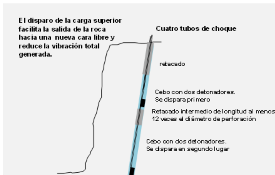
Figura 79: Cargas partidas en un barreno para reducir la carga operante (MIC)
