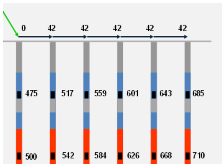
Figura 57: Esquema de secuenciación de una pega con cargas partidas, usando detonadores en fondo (475/500) y conectores en superficie de 42 ms.
