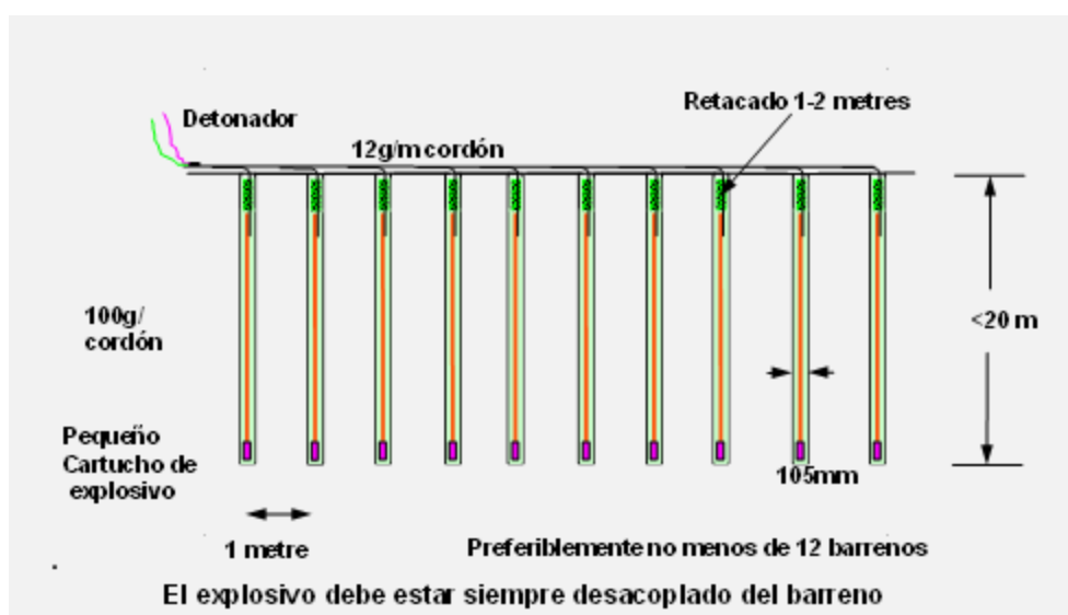
Figura 63: Carga de barrenos de precorte con cordón detonante
