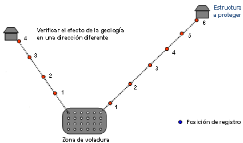
Figura 38: Disposición de sismógrafos en una zona de voladuras
