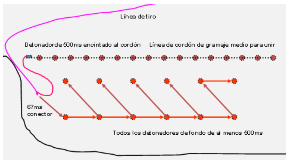
Figura 62: Esquema de precorte
