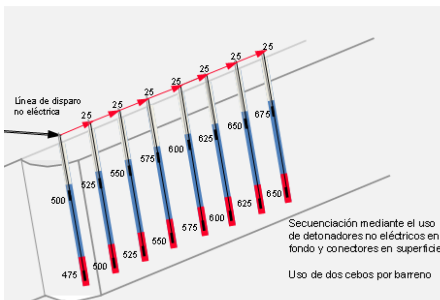
Figura 29: Secuencia de pega no eléctrica con dos detonador por barreno (475 ms/500 ms) y conectores de 25 ms en superficie
