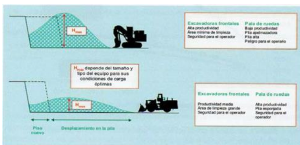
Figura 36: Consideraciones sobre la forma requerida de la pila de material en función de la maquinaria disponible
