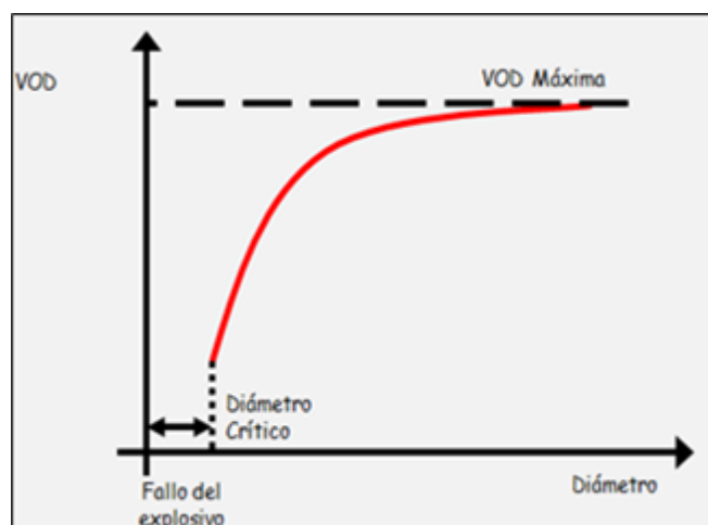
Figura 4: Relación entre el diámetro de carga y la VOD
