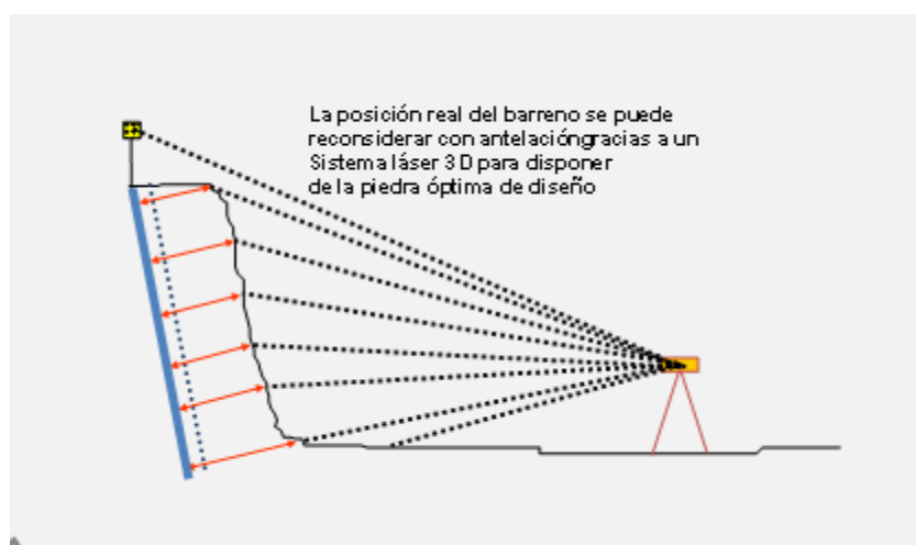
Figura 45: Replanteamiento de la posición del barreno para adaptarse a la piedra de diseño
