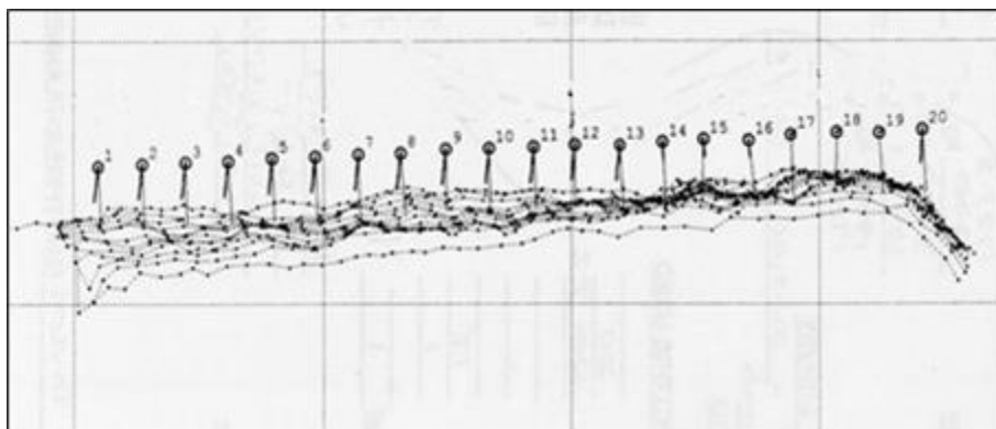
Figura 43: Vista real en planta de una perforación en banco, obtenida mediante láser 3D y sonda de medición de barrenos
