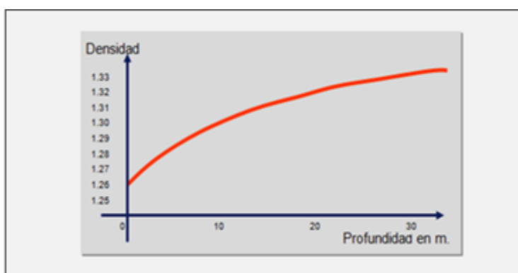
Figura 2: Ejemplo de la variación de la densidad de una emulsión ( \text{g/cm}^3 ) con la profundidad del barreno
