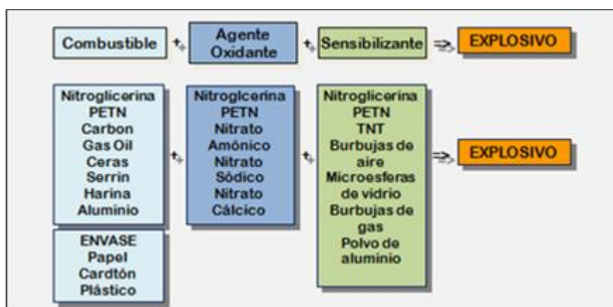
Figura 1: Componentes de un explosivo
