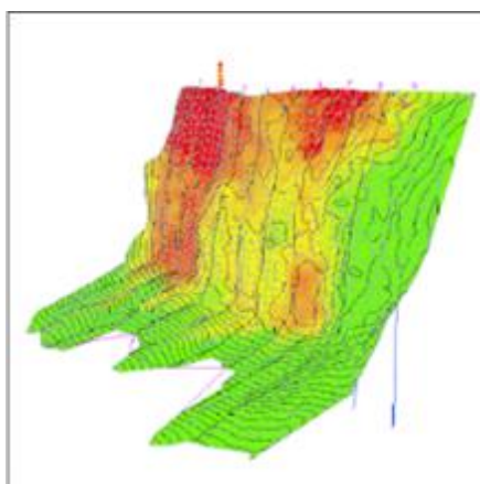
Figura 39: Modelo tridimensional de un frente de voladura
