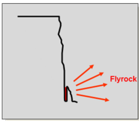
Figura 66: Proyecciones generadas por el disparo de un barreno corto en el pie del banco
