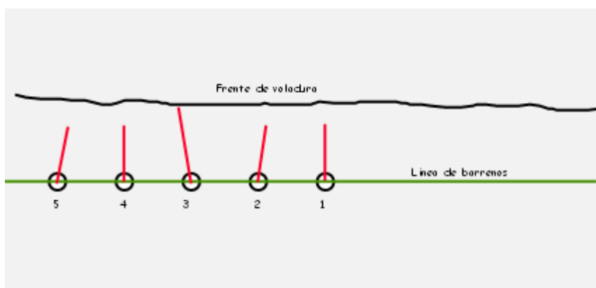
Figura 41: Influencia del azimut en el espaciamiento entre barrenos
