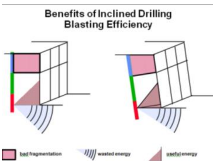
Figura 52: Aprovechamiento de la energía del explosivo en barrenos inclinados
