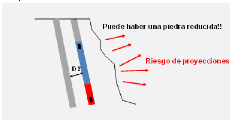
Figura 76: Esquema de perforación de un barreno paralelo
