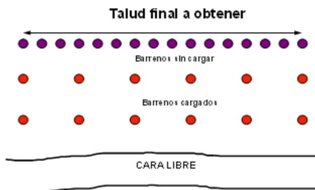
Figura 61: Barrenos vacíos
