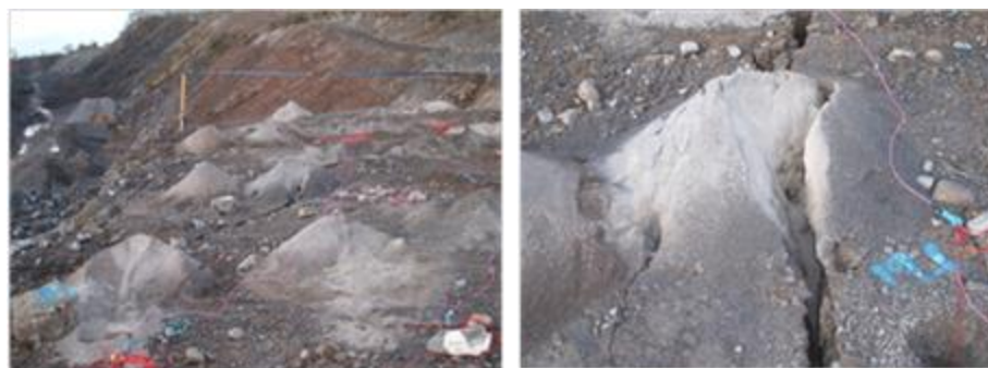
Figura 75: Movimiento que indica la presencia de barrenos fallidos
