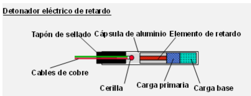
Figura 13: Esquema de un detonador eléctrico
