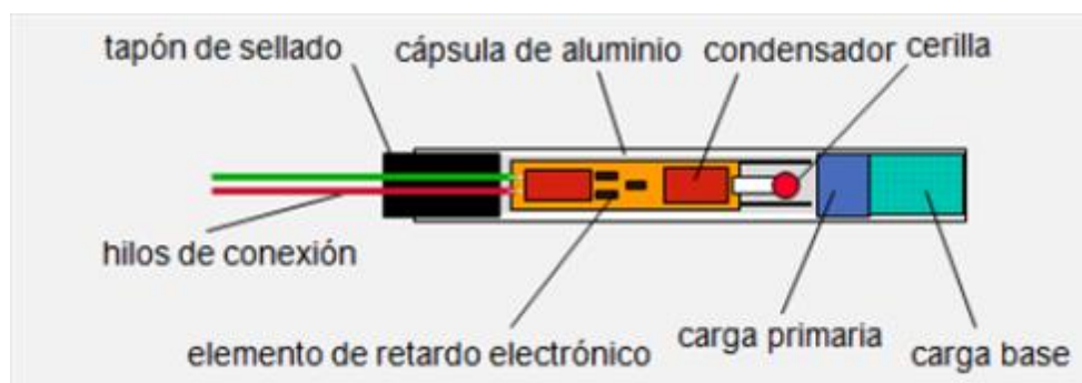
Figura 17: Detonador electrónico
