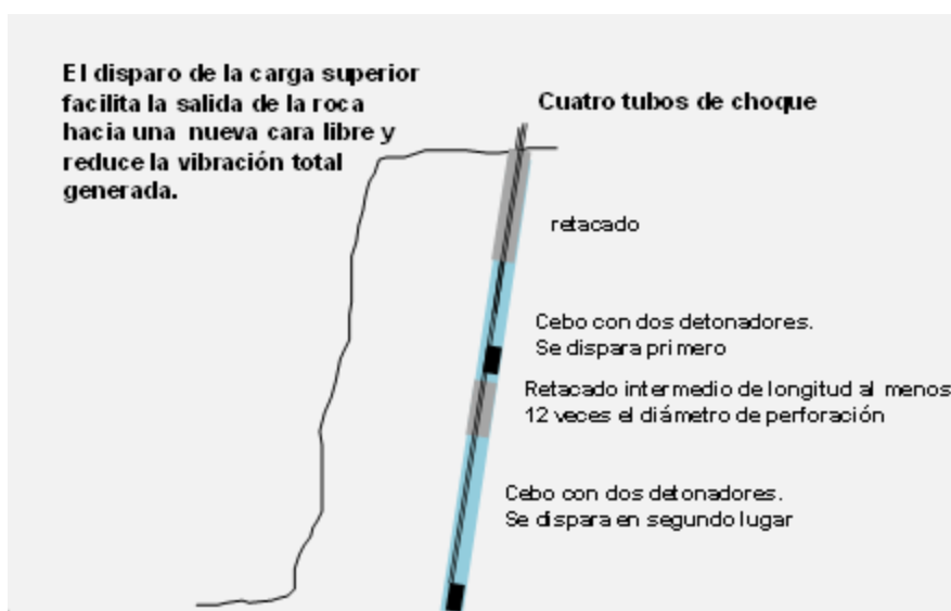
Figura 53: Disposición de carga y secuenciación en barrenos con cargas partidas
