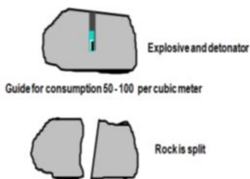
Figura 58: Taqueo de un bloque mediano mediante el disparo de un barreno en él
