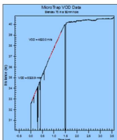
Figura 3: Medición de la velocidad de detonación de una mezcla a granel de emulsión - anfo de un barreno de 92 mm
