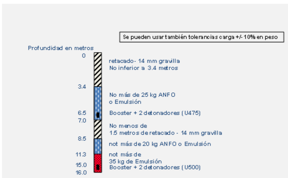
Figura 72: Ejemplo de un diagrama de carga
