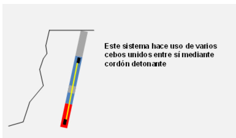
Figura 25: Posible esquema híbrido de iniciación de un barreno haciendo uso de cordón y cebos
