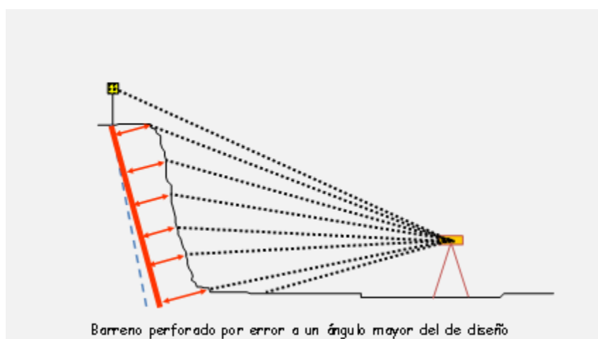
Figura 40: Errores en el ángulo de perforación. Variación de la distancia real a la cara libre
