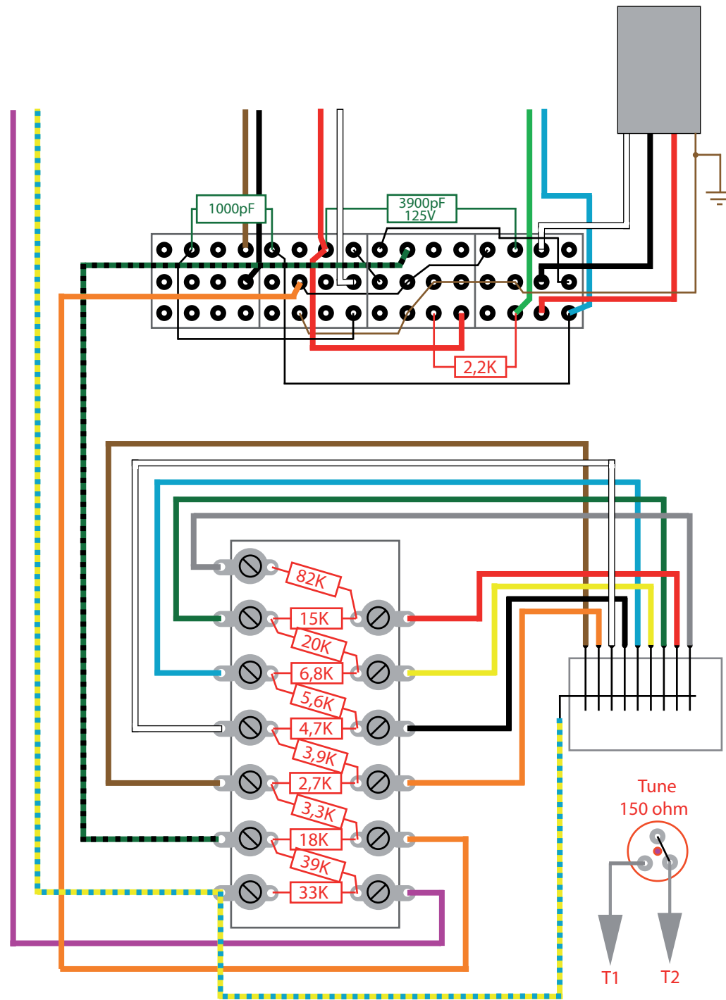
Platine commande
