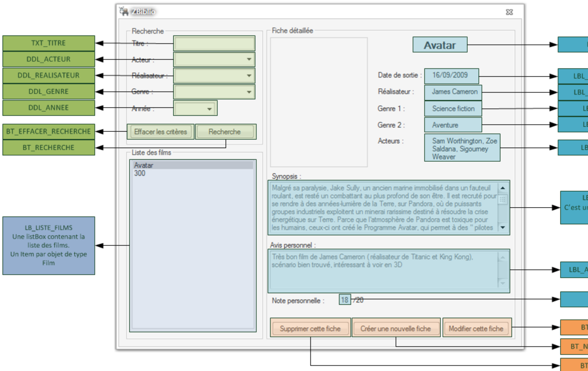
Fenêtre principale. Name : ZBiblio
