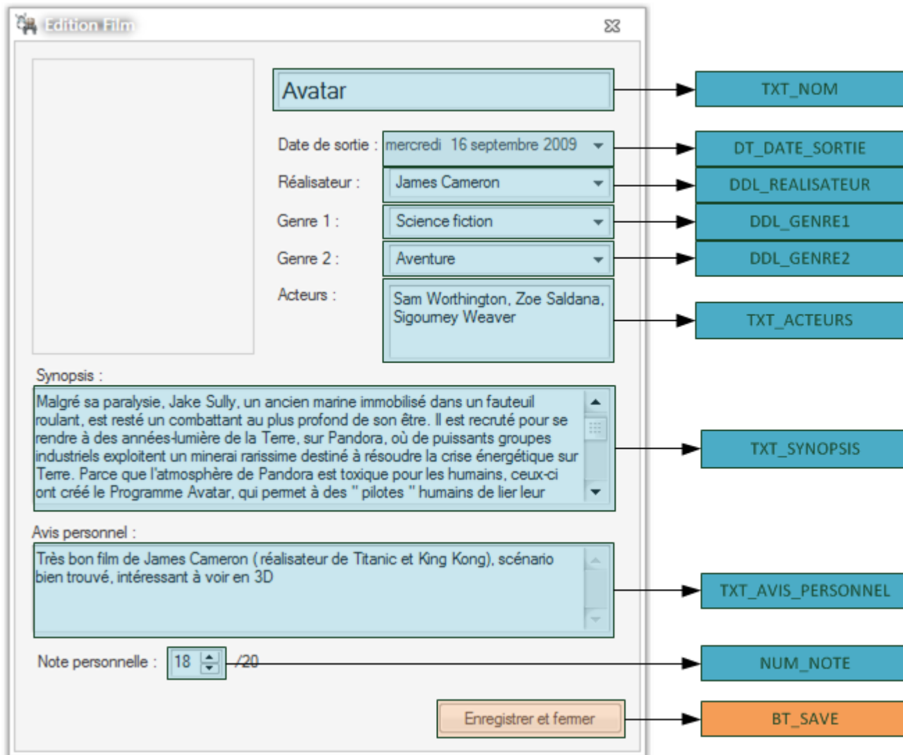
Fenêtre d'ajout/modification. Name : AjoutEditionFilm
