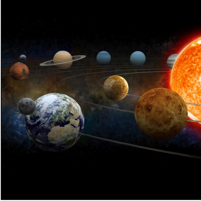
systeme solaire
