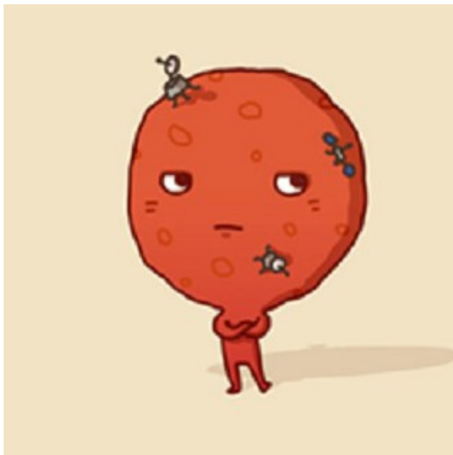
mars
