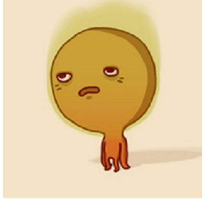
vénus
