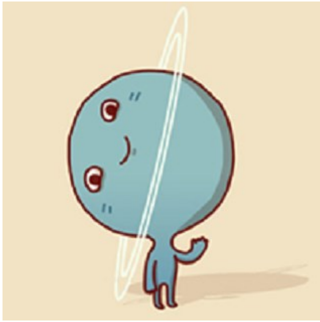
uranus
