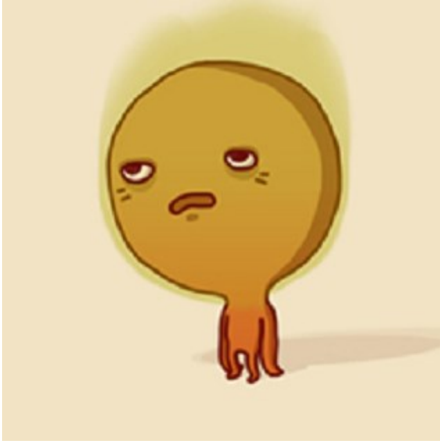
vénus
