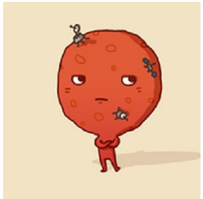
mars
