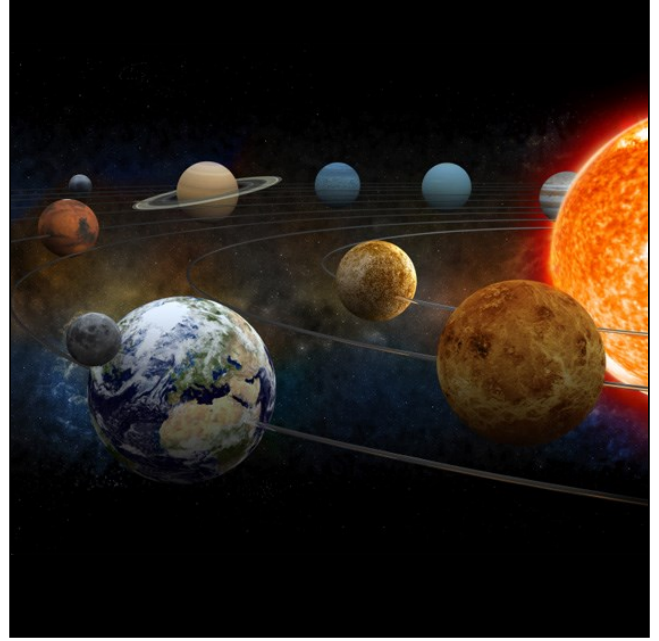
systeme solaire
