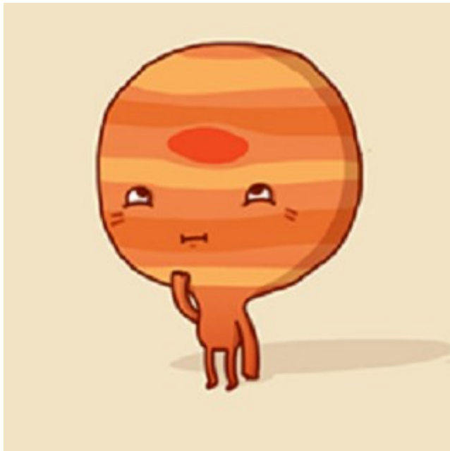
jupiter
