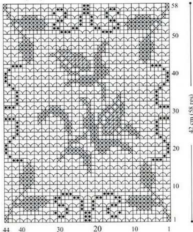
motif B (10 fs)
