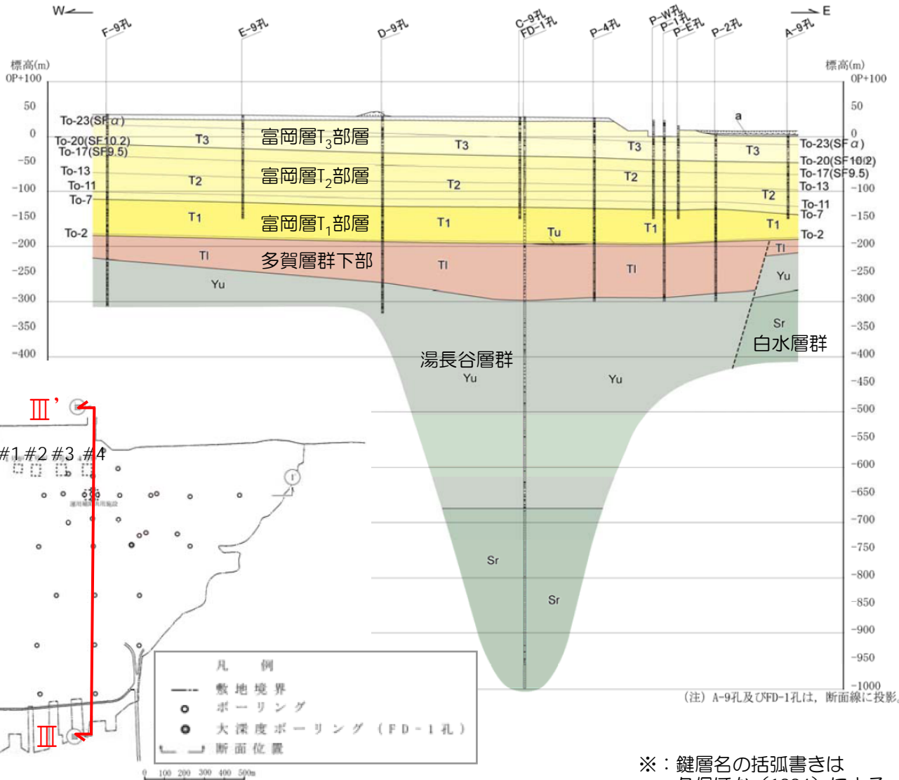
地質断面図 (Ⅲ-Ⅲ' 断面)
